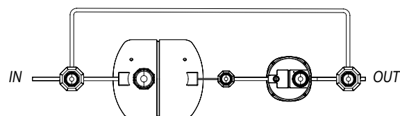
schema indicativo
