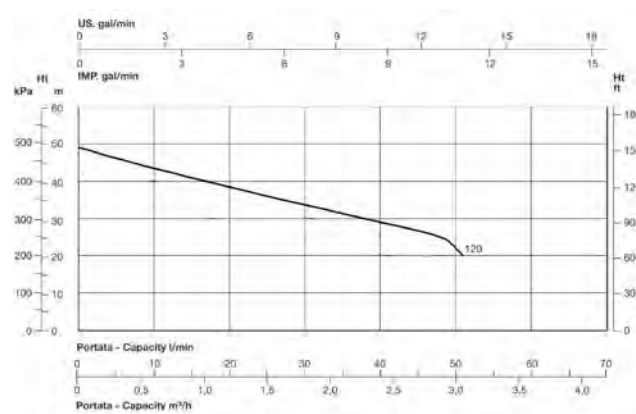
Caratteristiche elettro-pompa
