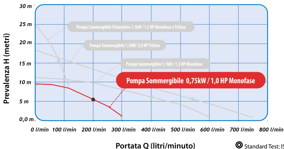
Pompa con girante VORTEX (arretrata) in Acciaio INOX AISI 304
