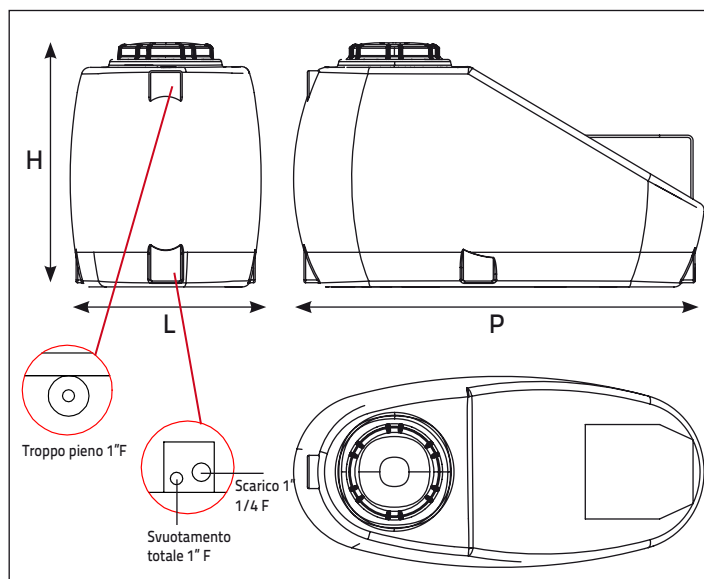
Serbatoio dotato di mensola per installazione Kit autoclave (non compreso)
