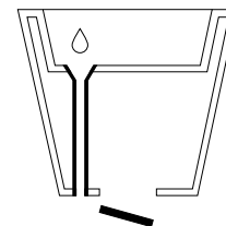
portavaso con sottotappo e sistema di drenaggio pot with insert, lid and drainage system
